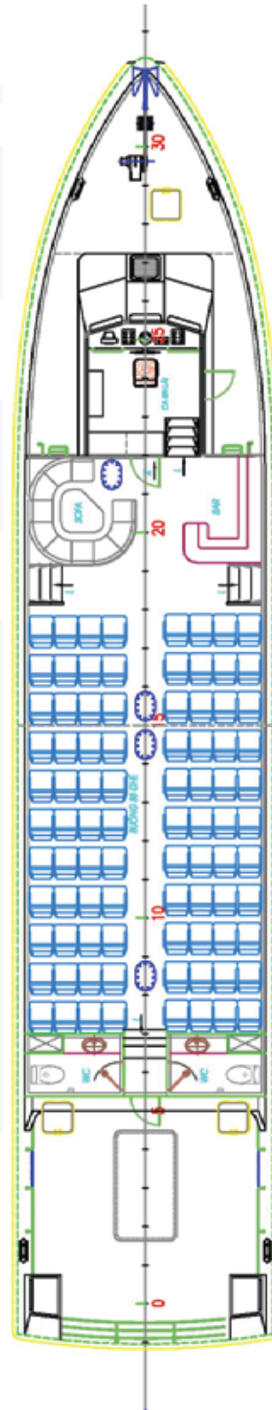
SƠ ĐỒ BỐ TRÍ GHẾ NGỒI TÀU K7 (96 khách)
